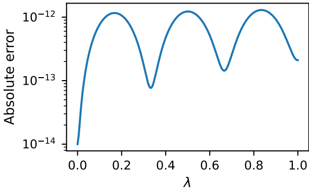
One-qubit VQE error
