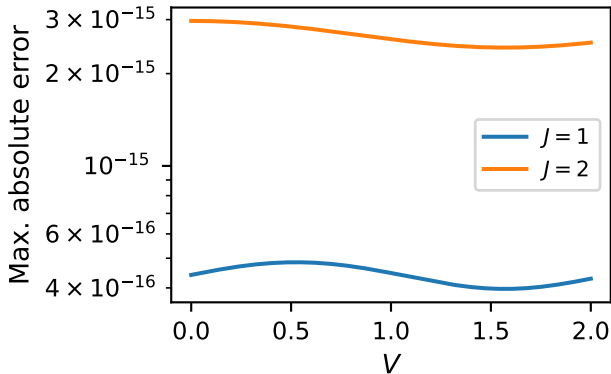
Lipkin VQE errors
