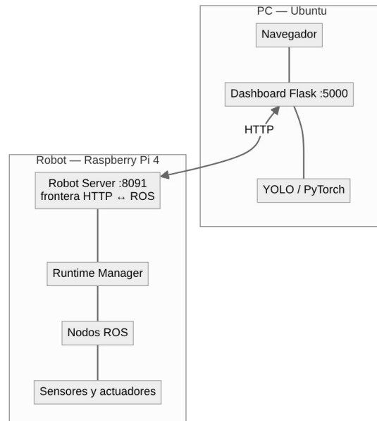
Figura 1. Arquitectura del sistema: computadora de control y robot.
