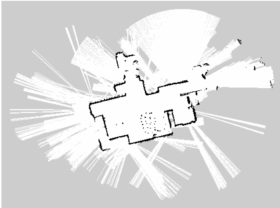
Figura 3. Mapa construido por el robot con SLAM (Gmapping).
