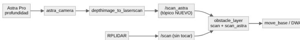
Diagrama 2. Opción A: la profundidad de la Astra Pro como segunda fuente del costmap, sin tocar /scan.
