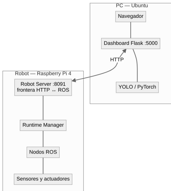
Diagrama 1. Arquitectura en tres capas: la PC y el robot, con el Robot Server como única frontera HTTP ↔ ROS.
