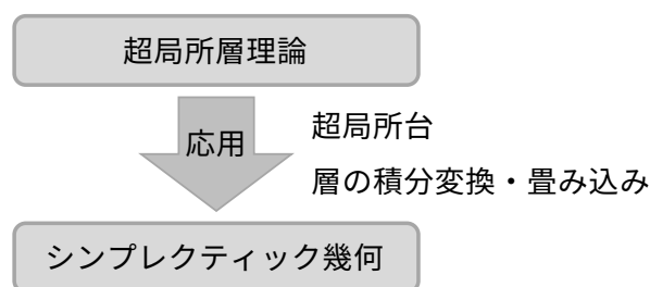
図1: 超局所層理論とシンプレクティック幾何
