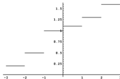
Рисунок — Вид функции распределения дискретной случайной величины \xi , принимающей лишь целые значения x = \dots, -3, -2, \dots, 2, 3, \dots . Скачки функции F_{\xi}(x) в целых точках x = \dots, -3, -2, \dots, 2, 3, \dots по величине равны соответствующим вероятностям P_{\xi}(x) .
