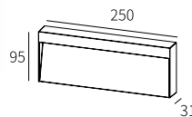
Dimension : 250x95x31
