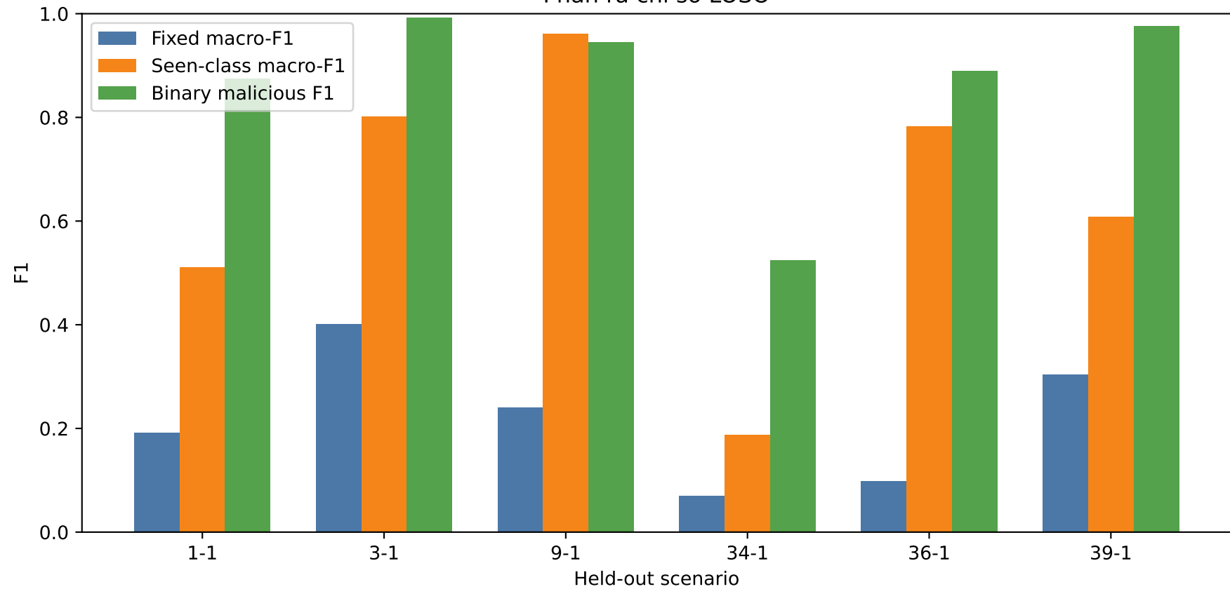
Phân rã chỉ số LOSO
