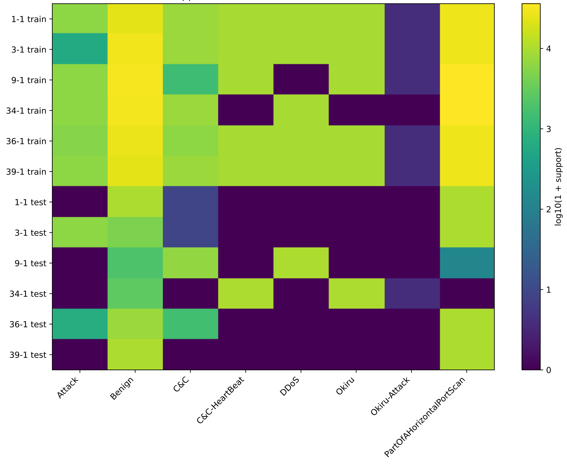
Support train/test theo class và LOSO fold
