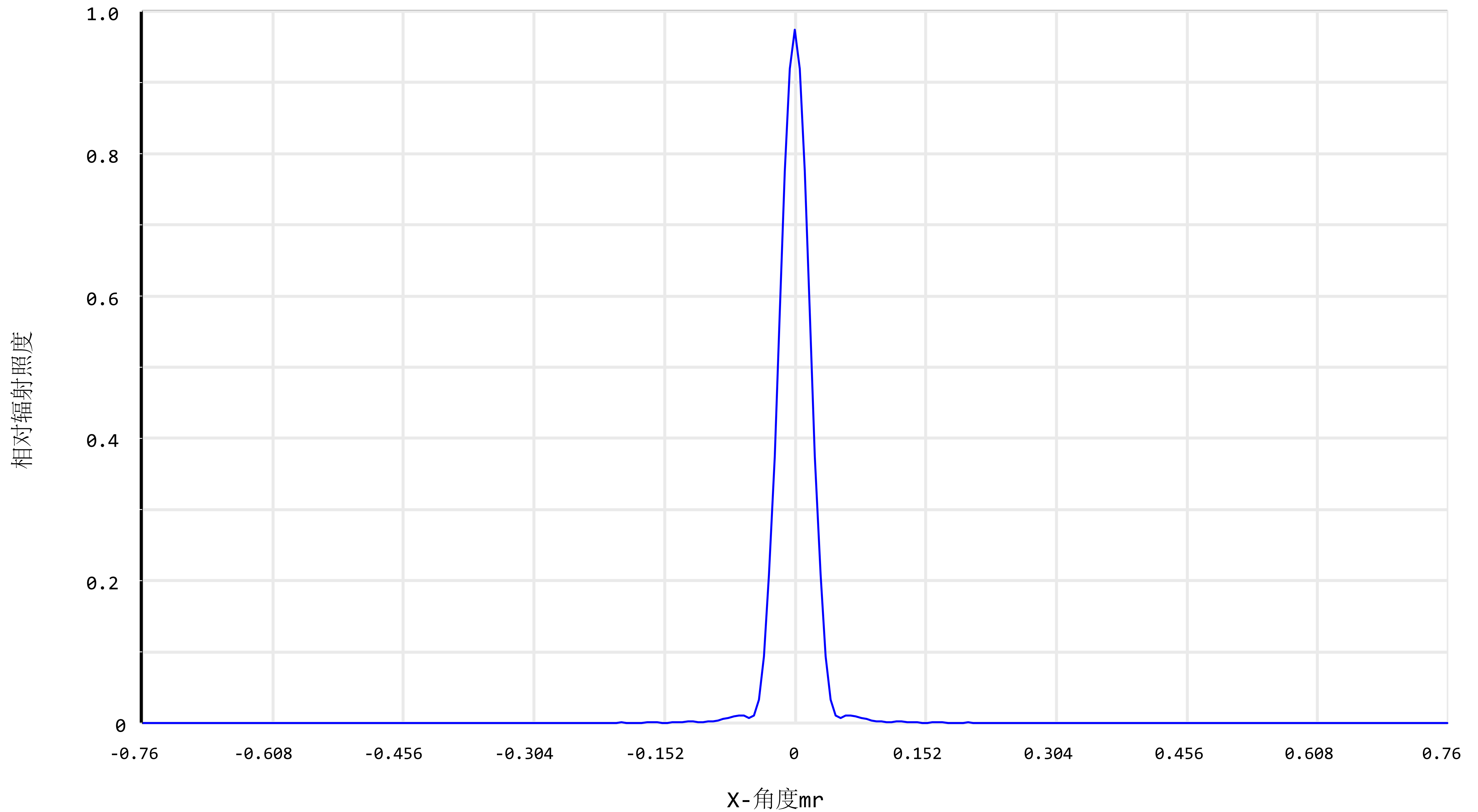
PSF截面图
