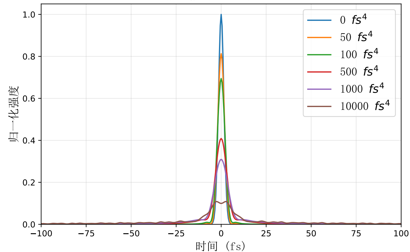
四阶色散对5fs脉冲的影响
