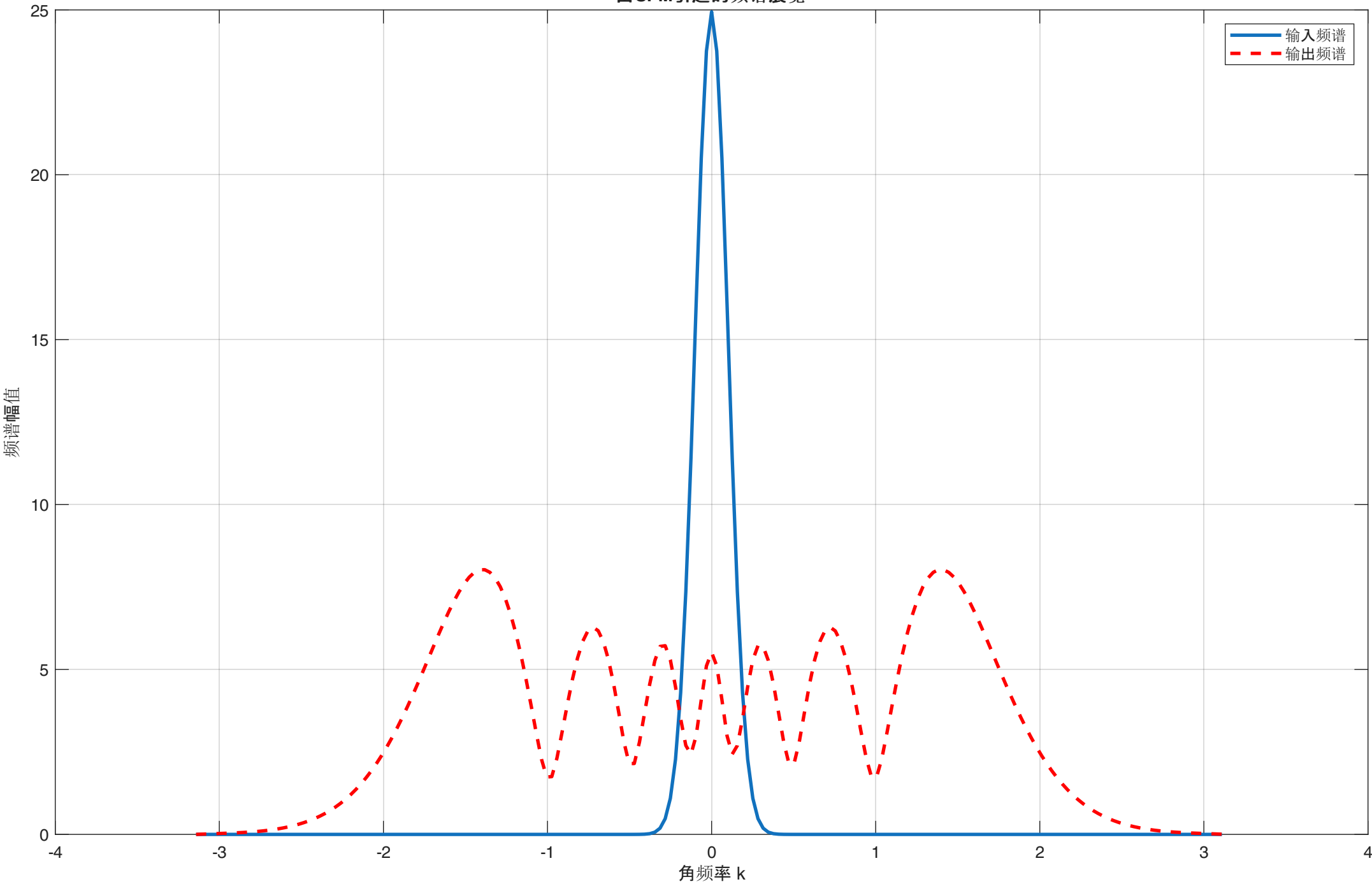
由SPM引起的频谱展宽
