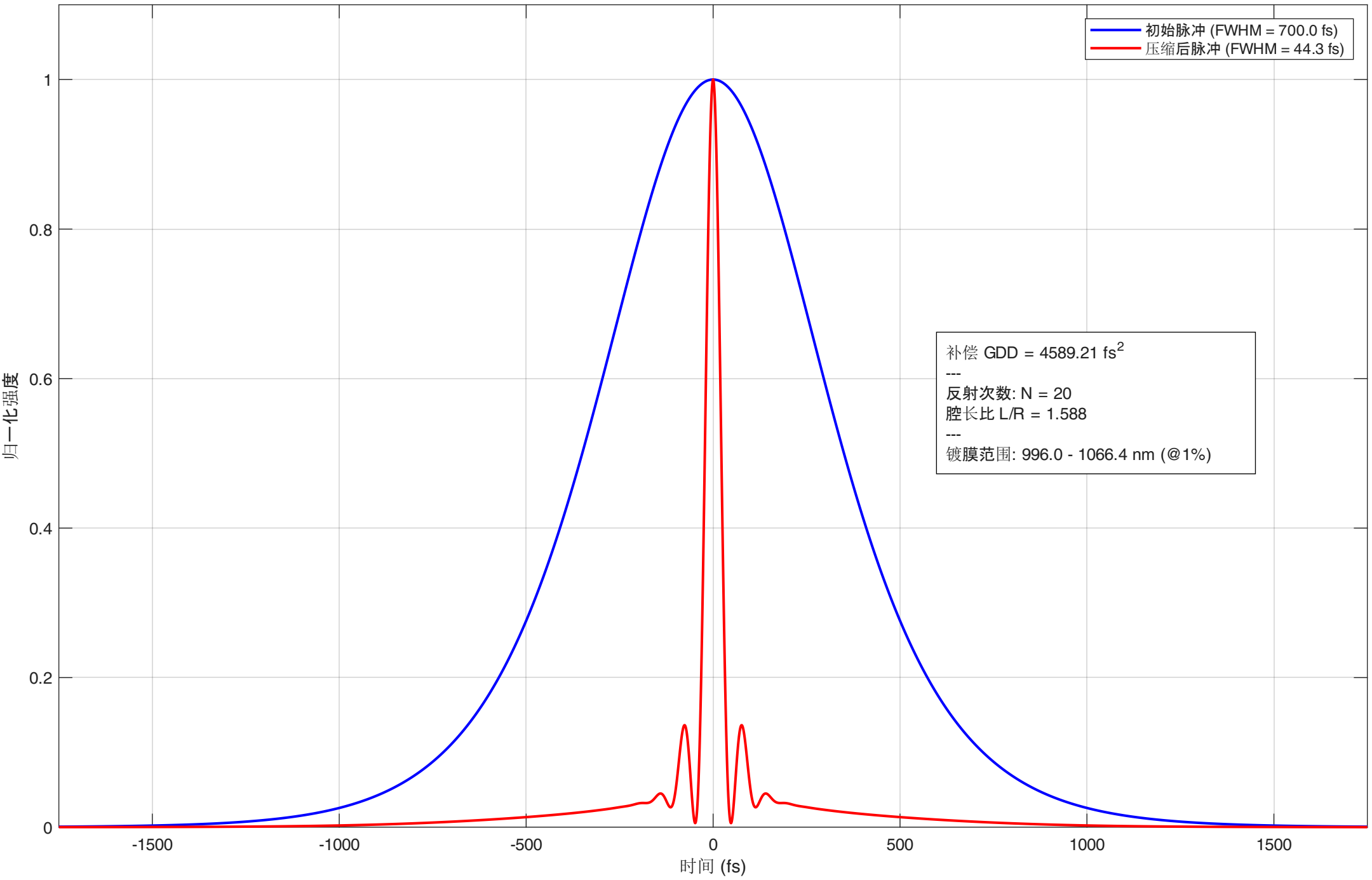
MPC 时域脉冲压缩 (脉冲能量: 500.00 uJ, 总 B 积分 \approx 24.25 rad)
