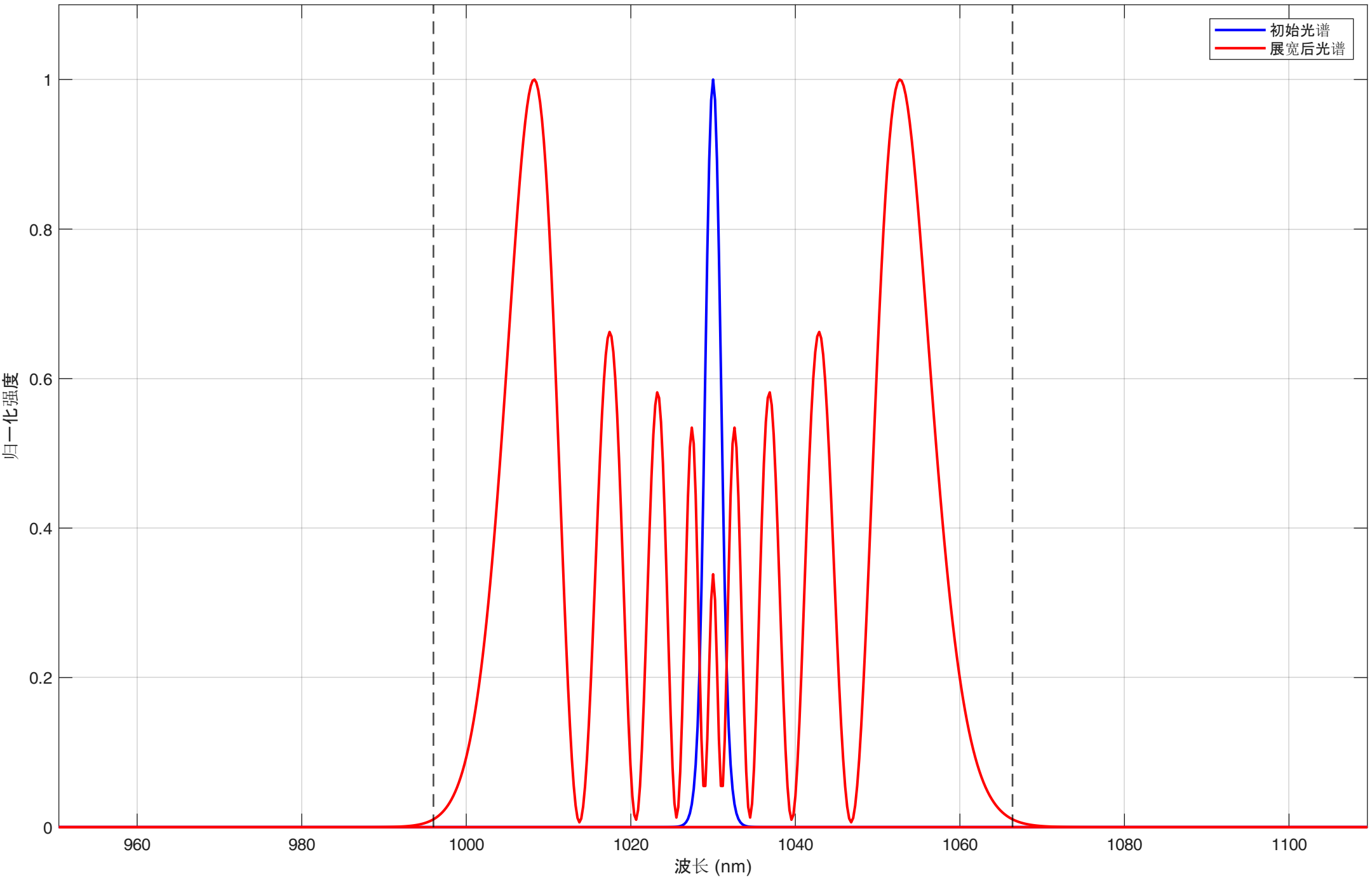
MPC 光谱展宽
