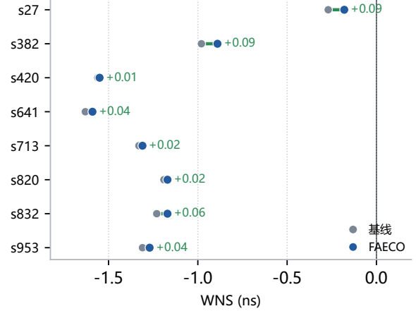
图 4 ISCAS89 顺序电路混合修复的基线与 FAECO 结果对比 (周期 0.5 ns; 标注为 FAECO 相对基线的 WNS 变化)
