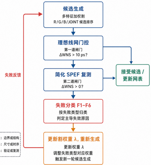
图 3 FAECO 失效驱动闭环与物理门控：启用物理门控时，候选先经理想线网与简化 SPEF 两道门控筛选，失败按 F1–F6 归类并更新割权重后重割
