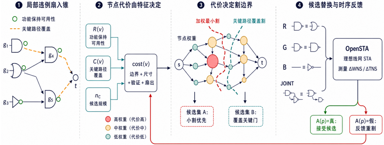
图 2 FAECO 机制原理：局部扇入锥中的特征决定节点代价，节点代价决定割边界，割边界生成等价候选并由 OpenSTA 反馈更新。
