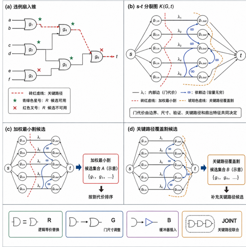
图 2 FAECO 候选构造与排序机制：加权最小割控制候选规模，关键路径覆盖割 C_c 补充时序关键候选，R 候选可用性参与策略切换；图中候选集合 A/B 分别对应 C_w 与 C_c 。
