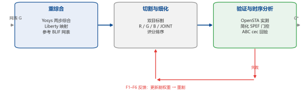
图 1 FAECO 三阶段流水线: 重综合 → 切割与细化 → 验证与时序分析。
