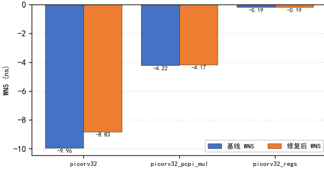
图 6: PicoRV32 异构基准的跨设计泛化
