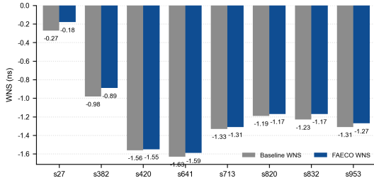
图 5 ISCAS89 顺序电路混合修复主结果（周期 0.5 ns）
