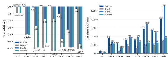
图 8 收敛配置竞争基线对比：左为修复后 WNS，右为候选 STA 调用次数
