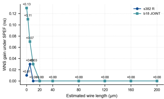
图 11 SPEF 负载扫描下 WNS 改善随线长的变化（s382 的 R 候选与 b18 的 JOINT 候选）
