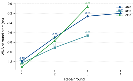
图 10 收敛配置下 WNS 随外环轮次收敛（每轮至多接受一个候选，数据点为轮开始时的网表 WNS）
