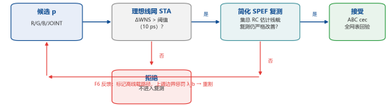
图 4 简化 SPEF 门控的两层验证流程：候选先经理想线网 OpenSTA 实测，改善超过阈值才进入简化 SPEF 复测，复测仍严格改善才接受；未通过者归类为 F6 反馈并上调边界惩罚后重割
