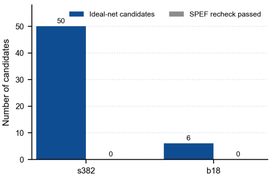
图 12 SPEF 门控复测：s382（50 个）与 b18（6 个）候选的复测通过数（当前 40 μm/unit 估计线载下全部未通过）
