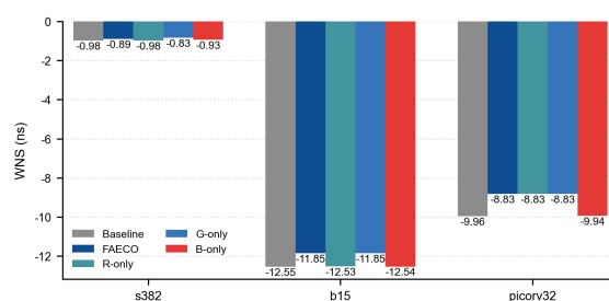
图 9 纯策略消融：基线、混合与纯 R/G/B 的最终 WNS (混合含 R/G/B/JOINT，窗口深度 3)
