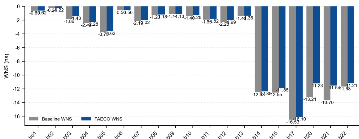
图 6 ITC-99 跨基准泛化：19 个可映射电路的 WNS 修复
