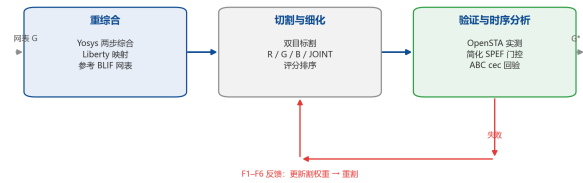
图 1 FAECO 三阶段流水线：重综合 → 切割与细化 → 验证与时序分析。
