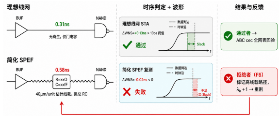
图 4 简化 SPEF 门控的两层验证流程: 候选先经理想线网 OpenSTA 实测, 改善超过阈值才进入简化 SPEF 复测, 复测仍严格改善才接受; 未通过者归类为 F6 反馈并上调边界惩罚后重割
