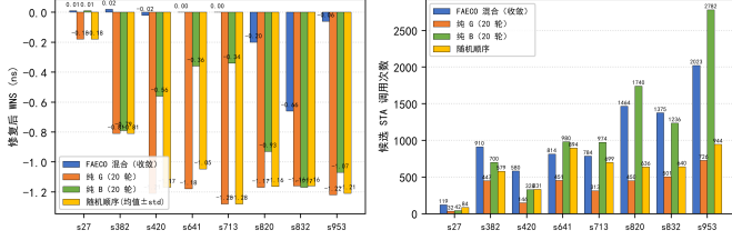
图 7. 收敛配置竞争基线对比（统一 OSS-CAD 0.67, 周期 0.5 ns, 均为 20 轮收敛语义）：左为修复后 WNS, 右为候选 STA 调用次数。
