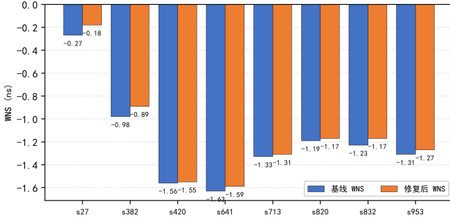
图 2. ISCAS89 顺序电路混合修复主结果(周期 0.5 ns;全部数据在统一 OSS-CAD 0.67 工具链下重生成;策略分布: JOINT 4 个(s27/s382/s420/s953)、G 3 个、R 1 个(s820))
