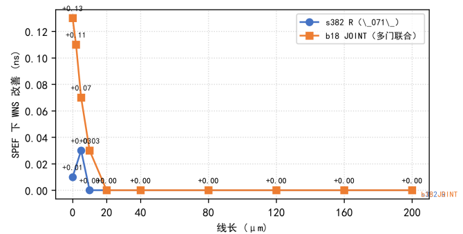
图 10. SPEF 负载扫描下 WNS 改善随线长的变化（s382 R 与 b18 JOINT）：两类候选均随估计线载增加衰减至归零，但 b18 JOINT 的轻负载保持区间更宽（2 \mu\text{m} 下 +0.11 ）。
