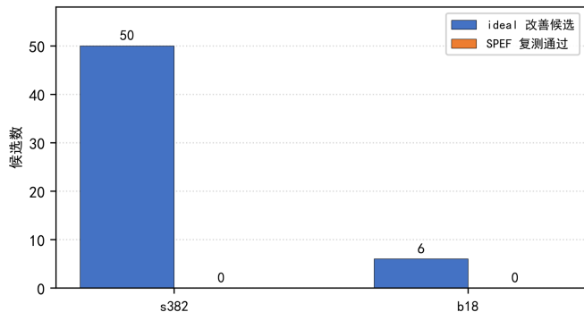
图 11. SPEF 门控的保守性初探：理想线网改善候选的 SPEF 复测通过数（统一 OSS-CAD 0.67 网表；纵轴为候选个数。当前 40\mu\text{m}/\text{unit} 估计线载下，s382 的 50 个与 b18 的 6 个候选全部未通过复测，反映门控参数偏保守而非修复失效；F6 反馈将边界惩罚从 1.0 逐轮提升到 6.0–7.0）
