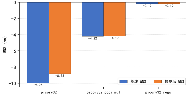
图 4. PicoRV32 异构基准 OOD 泛化 (统一 OSS-CAD 0.67 映射 + OpenSTA 实测, 周期见各电路)
