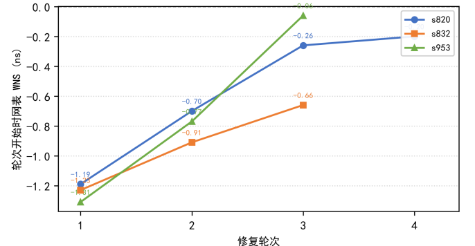
图 9. 收敛配置下 WNS 随轮次收敛（三个代表性电路；“轮”为 Algorithm 1 的外环 repeat 迭代——每轮对刷新后的关键路径实例逐一实测、每个实例至多接受一个候选，数据点为该轮开始时的网表 WNS，某轮无候选被接受即终止；统一 OSS-CAD 0.67，周期 0.5 ns；20 轮收敛语义）
