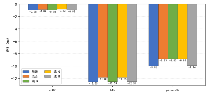
图 8. 纯策略消融（统一 OSS-CAD 0.67，周期 0.5ns / picorv32 5.0ns；混合 = R,G,B 全开；括号内为接受的候选类型）
