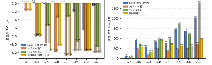
图 7. 收敛配置竞争基线对比（统一 OSS-CAD 0.67，周期 0.5 ns，均为 20 轮收敛语义）：左为修复后 WNS，右为候选 STA 调用次数。
