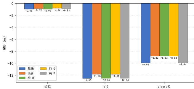
图 8. 纯策略消融（统一 OSS-CAD 0.67，周期 0.5 ns / picorv32 5.0 ns；混合 = R,G,B 全开；括号内为接受的候选类型）
