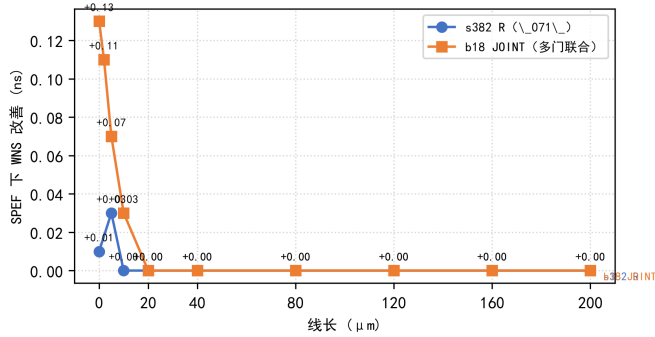
图 10. SPEF 负载扫描下 WNS 改善随线长的变化 (s382 R 与 b18 JOINT)
