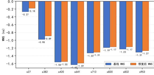
图 2. ISCAS89 顺序电路混合修复主结果 (周期 0.5 ns)
