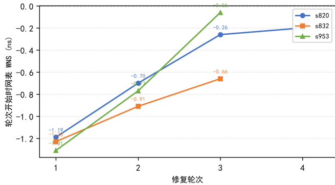
图 9. 收敛配置下 WNS 随轮次收敛（三个代表性电路；“轮”为 Algorithm 1 的外环迭代，每轮至多接受一个候选，数据点为该轮开始时网表 WNS）
