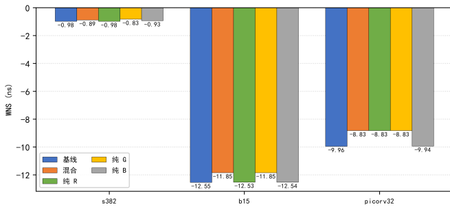
图 8. 纯策略消融（混合 = R/G/B 全开；括号内为接受的候选类型）
