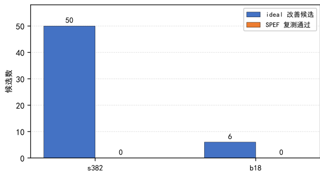
图 11. SPEF 门控的保守性初探：理想线网改善候选的 SPEF 复测通过数 (当前 40 μm/unit 估计线载下, s382 的 50 个与 b18 的 6 个候选全部未通过复测, 反映门控参数偏保守而非修复失效)
