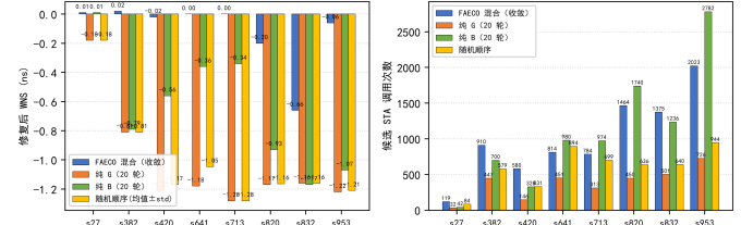
图 7. 收敛配置竞争基线对比：左为修复后 WNS，右为候选 STA 调用次数
