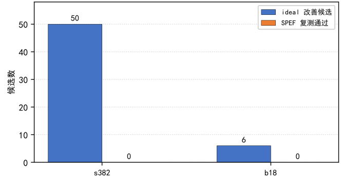
图 11. SPEF 门控的保守性初探：理想线网改善候选的 SPEF 复测通过率（当前 40\mu\text{m}/\text{unit} 估计线载下，s382 的 50 个与 b18 的 6 个候选全部未通过复测，反映门控参数偏保守而非修复失效）
