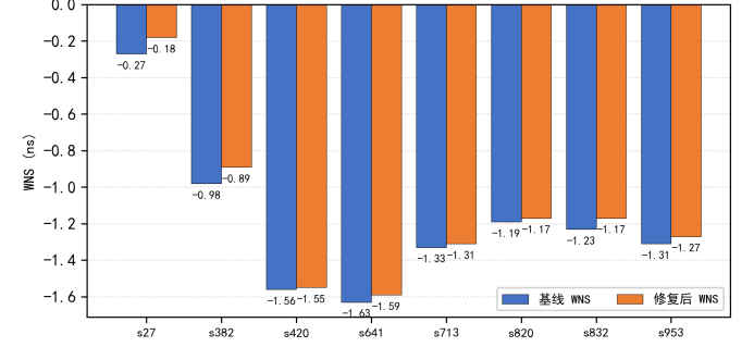
图 2. ISCAS89 顺序电路混合修复主结果 (周期 0.5 ns)
