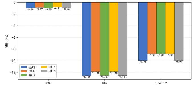
图 8. 纯策略消融：基线、混合与纯 R/G/B 的最终 WNS（混合含 R/G/B/JOINT，窗口深度 3）
