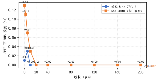
图 10. SPEF 负载扫描下 WNS 改善随线长的变化（s382 的 R 候选与 b18 的 JOINT 候选）
