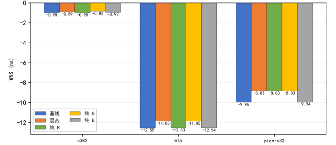
图 8. 纯策略消融：基线、混合与纯 R/G/B 的最终 WNS（混合含 R/G/B/JOINT，窗口深度 3）
