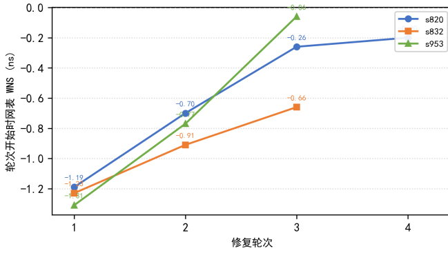
图 7: 收敛配置下 WNS 随轮次收敛 (三个代表性电路; “轮”为算法 1 的外环迭代, 每轮至多接受一个候选, 数据点为该轮开始时网表 WNS)
