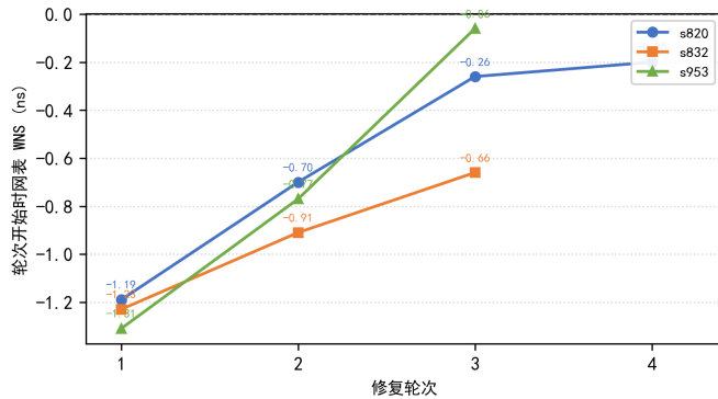
图 7: 收敛配置下 WNS 随轮次收敛（三个代表性电路；“轮”为算法 1 的外环迭代，每轮至多接受一个候选，数据点为该轮开始时网表 WNS）
