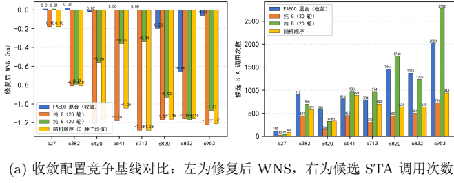
(a) 收敛配置竞争基线对比：左为修复后 WNS，右为候选 STA 调用次数
