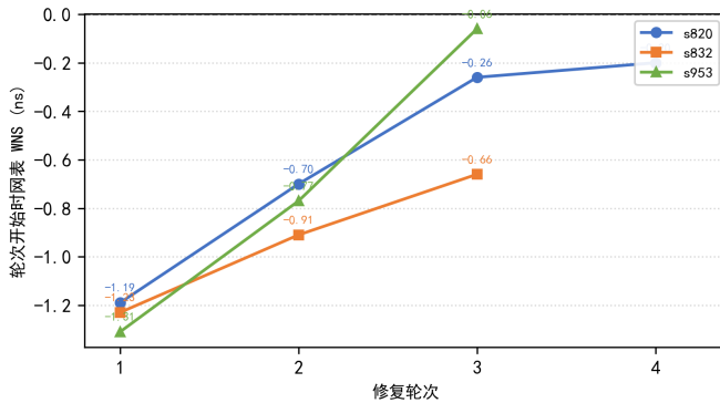
图 9: 收敛配置下 WNS 随轮次收敛，三个代表性电路的轮次为算法 1 的外环迭代，每轮至多接受一个候选，数据点为该轮开始时网表 WNS
