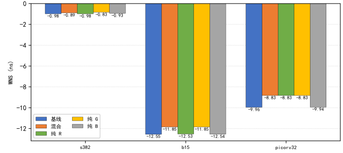
(b) 纯策略消融：基线、混合与纯 R/G/B 的最终 WNS (混合含 R/G/B/JOINT, 窗口深度 3)
