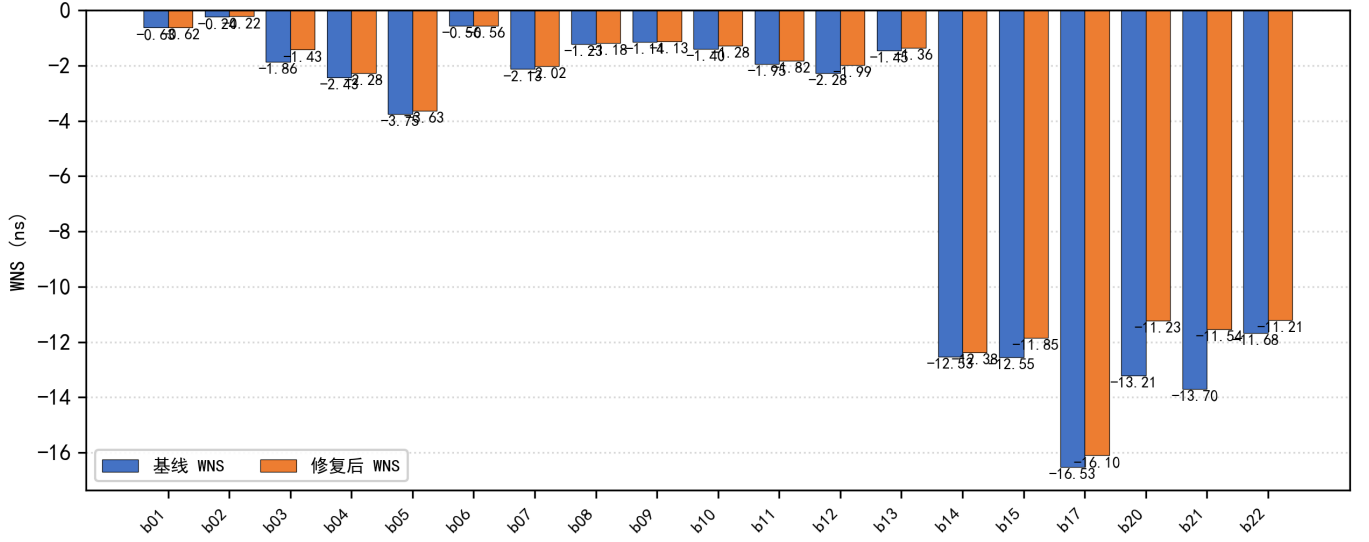
图 5: ITC-99 跨基准泛化: 19 个可映射电路的 WNS 修复
