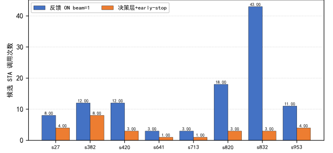
图 8: 轮内决策与提前停止的 STA 效率
