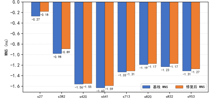
图 4: ISCAS89 顺序电路混合修复主结果 (周期 0.5 ns)
