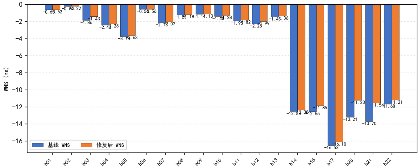
图 5: ITC-99 跨基准泛化: 19 个可映射电路的 WNS 修复
