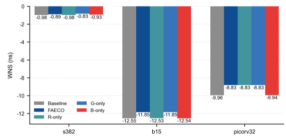
图 9 纯策略消融：基线、混合与纯 R/G/B 的最终 WNS (混合含 R/G/B/JOINT，窗口深度 3)
