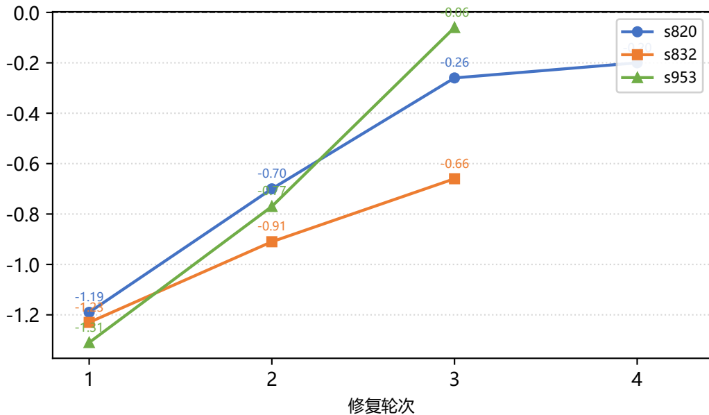
轮次开始时网表 WNS (ns)
