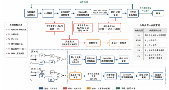
图 3 FAECO 失效驱动闭环与物理门控：启用物理门控时，候选先经理想线网与简化 SPEF 两道门控筛选，失败按 F1-F6 归类并更新割权重后重割
