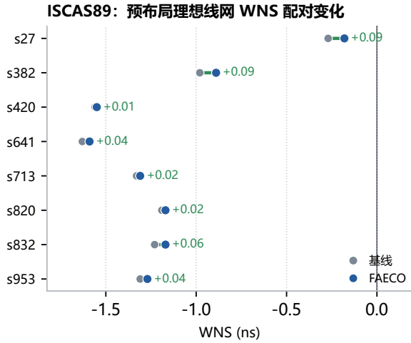
图 4 ISCAS89 顺序电路混合修复的基线与 FAECO 结果对比 (周期 0.5 ns; 标注为 FAECO 相对基线的 WNS 变化)
