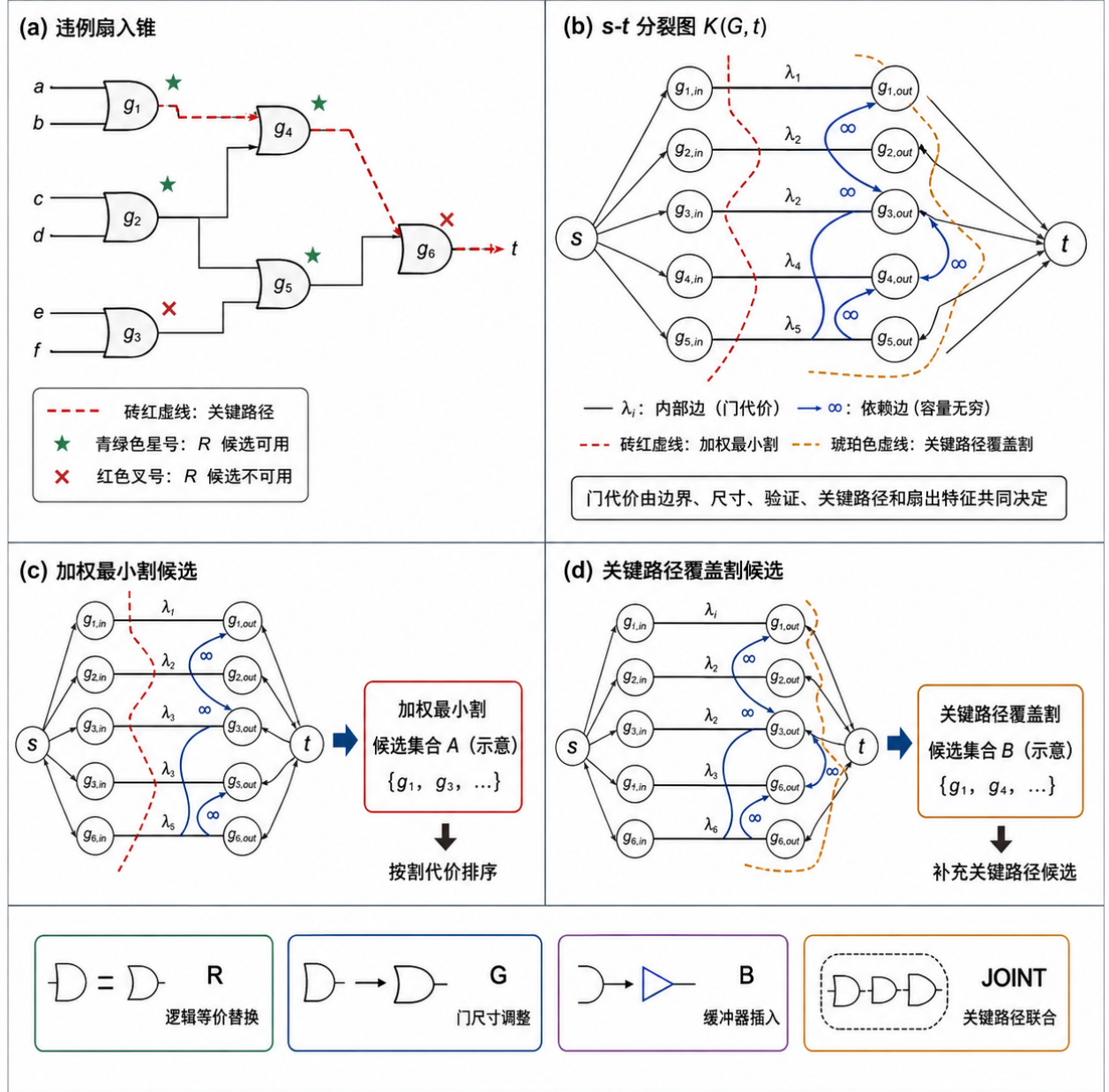
图 2 FAECO 机制原理：局部扇入锥中的特征决定节点代价，节点代价决定割边界，割边界生成等价候选并由 OpenSTA 反馈更新。
