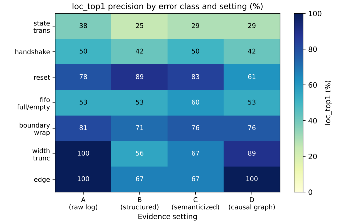
图 3. 错误类别 × 设置的定位 Top-1 精度热力图。困难类别排序 (状态迁移/握手低于位宽截断/边沿) 在全部设置中成立。
