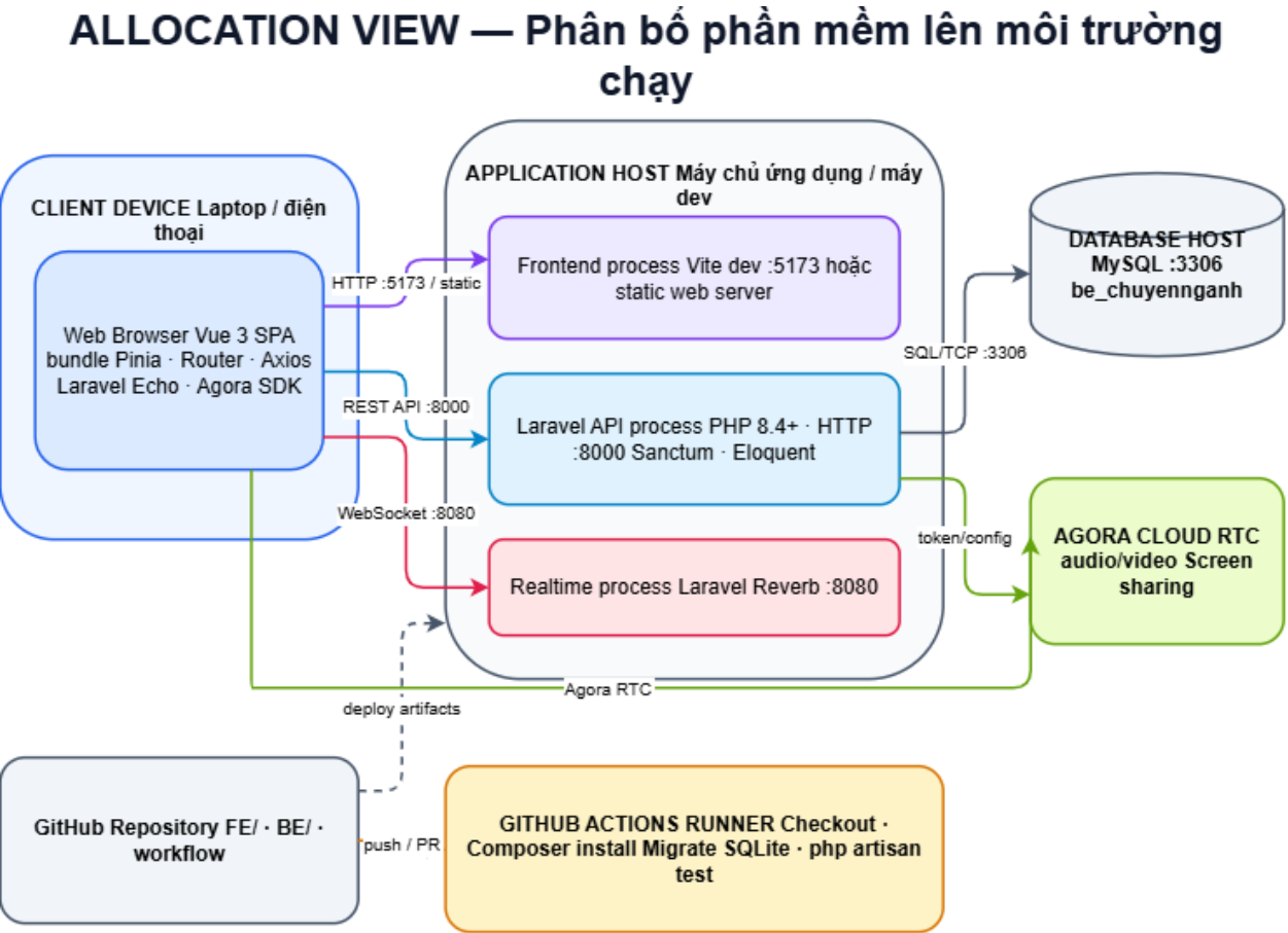
Hình 7: Allocation View
