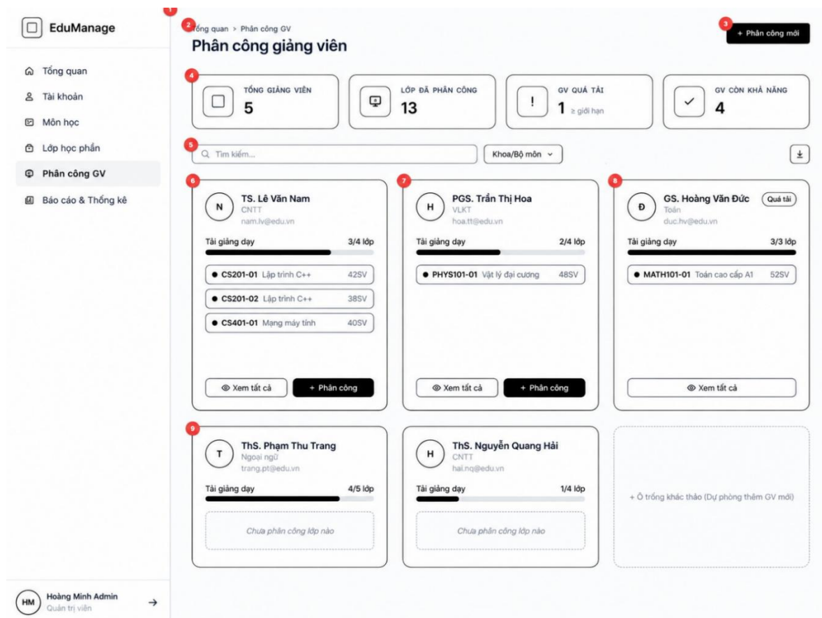
Hình 2.16.1 Giao diện phân công giảng dạy
