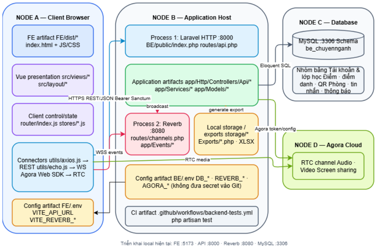
Hình 6.2: Detailed Allocation View
