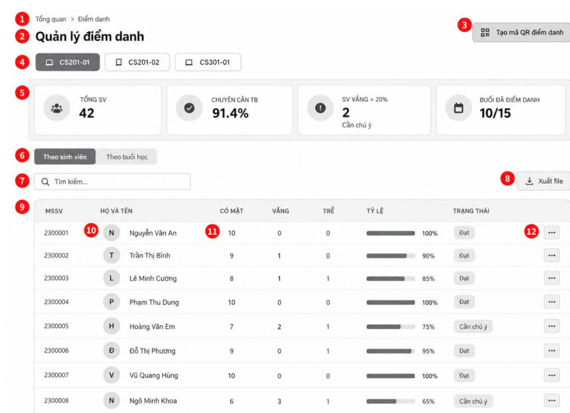
Hình 2.10.1 Giao diện quản lý điểm danh
