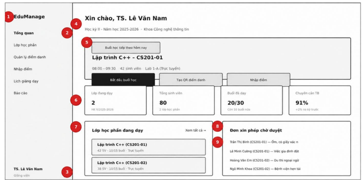
Hình 2.2.2 Giao diện Dashboard giảng viên
