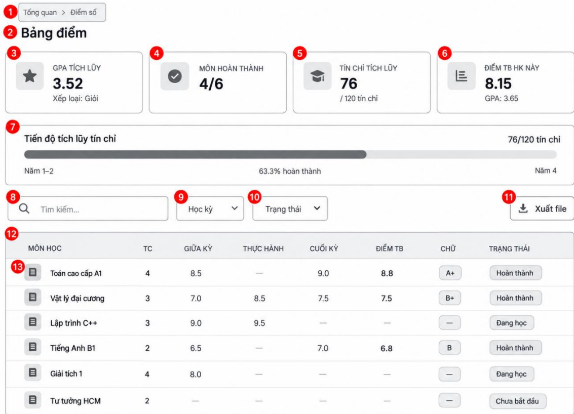
Hình 2.14.1 Giao diện bảng điểm
