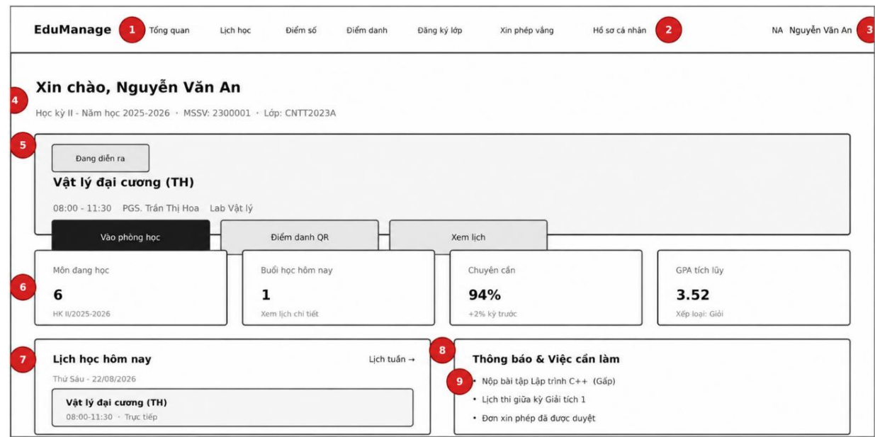
Hình 2.2.1 Giao diện Dashboard sinh viên
