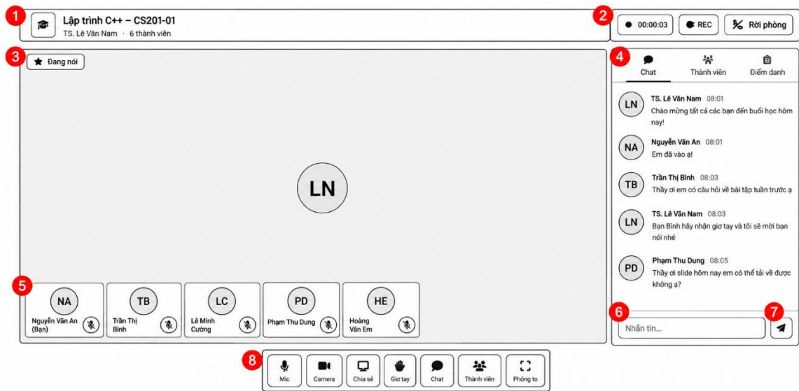
Hình 2.8.1. Giao diện phòng học trực tuyến
