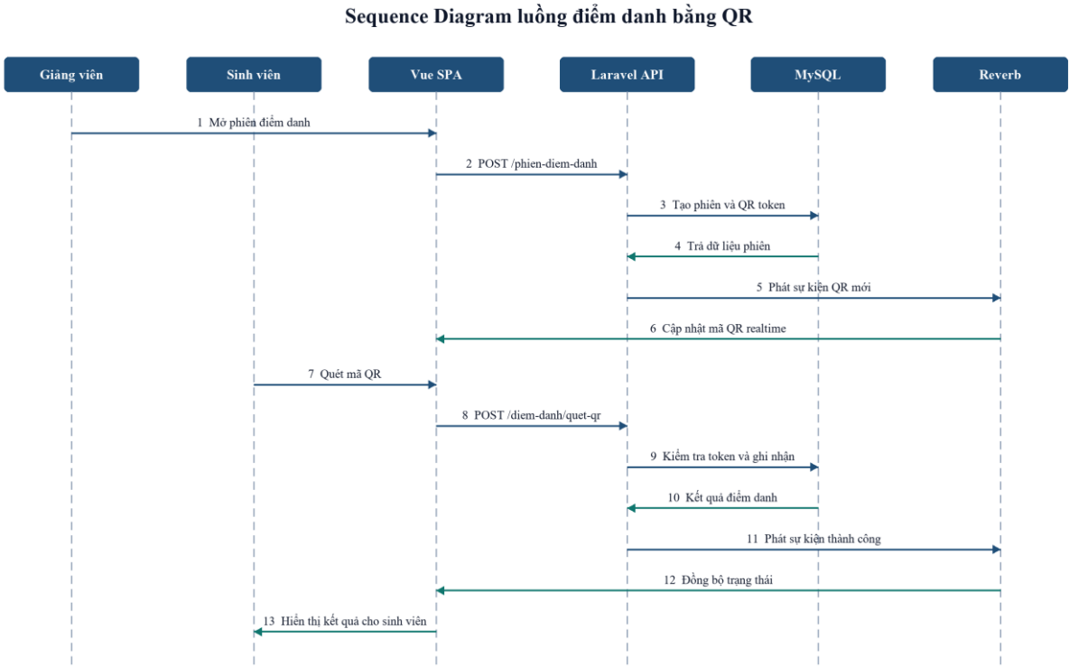
Hình 5.4: Biểu đồ tuần tự (Sequence Diagram) luồng điểm danh bằng QR
