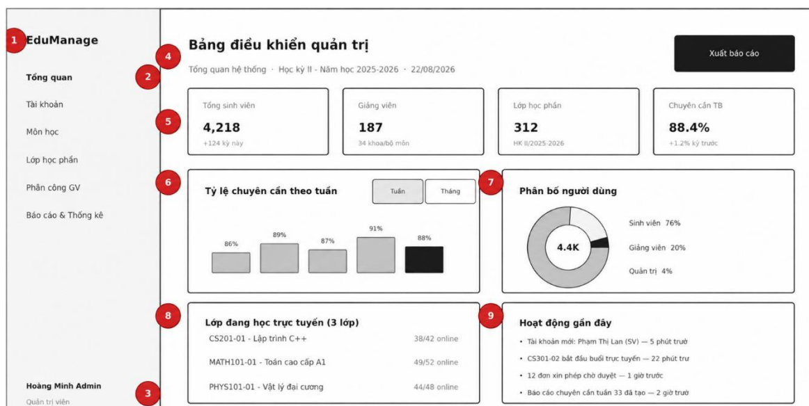
Hình 2.2.3. Giao diện Dashboard Admin
