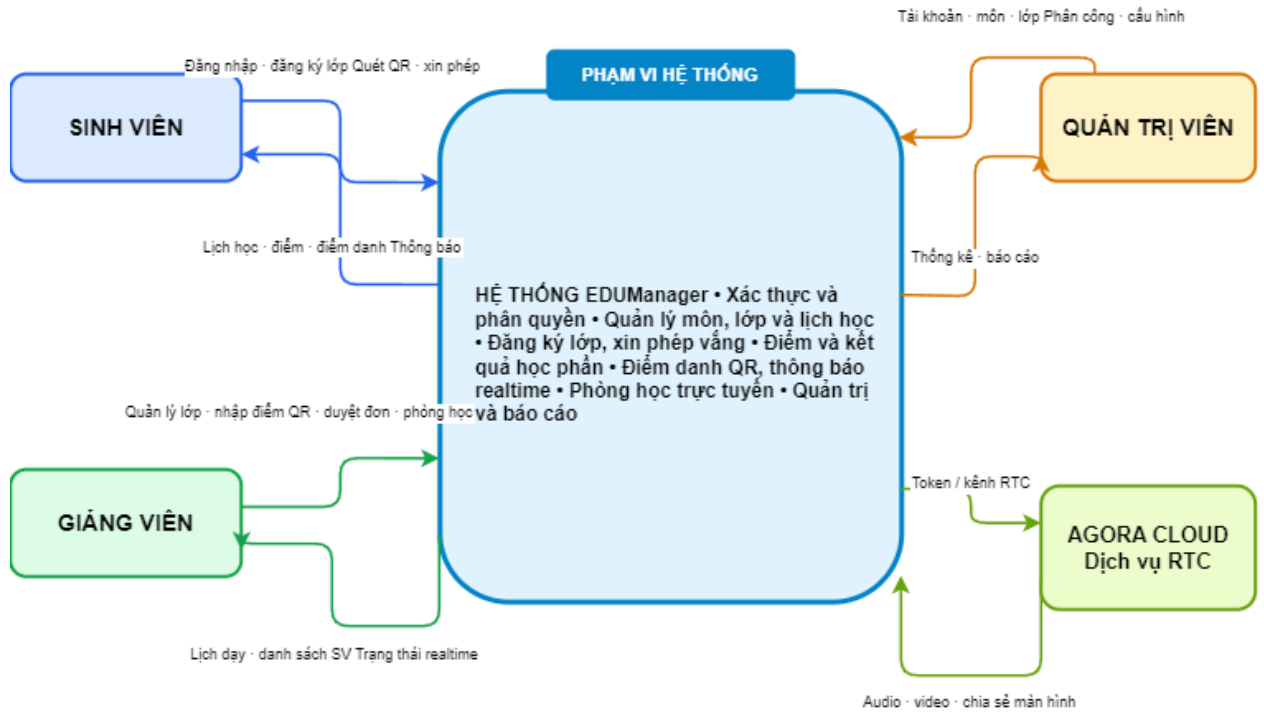
Hình 2.1: Sơ đồ ngữ cảnh của hệ thống
