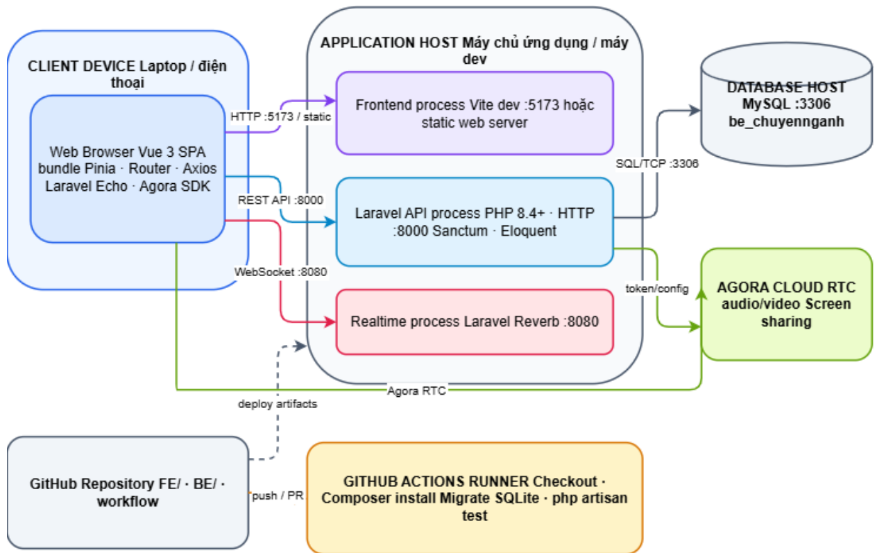
Hình 7: Allocation View
