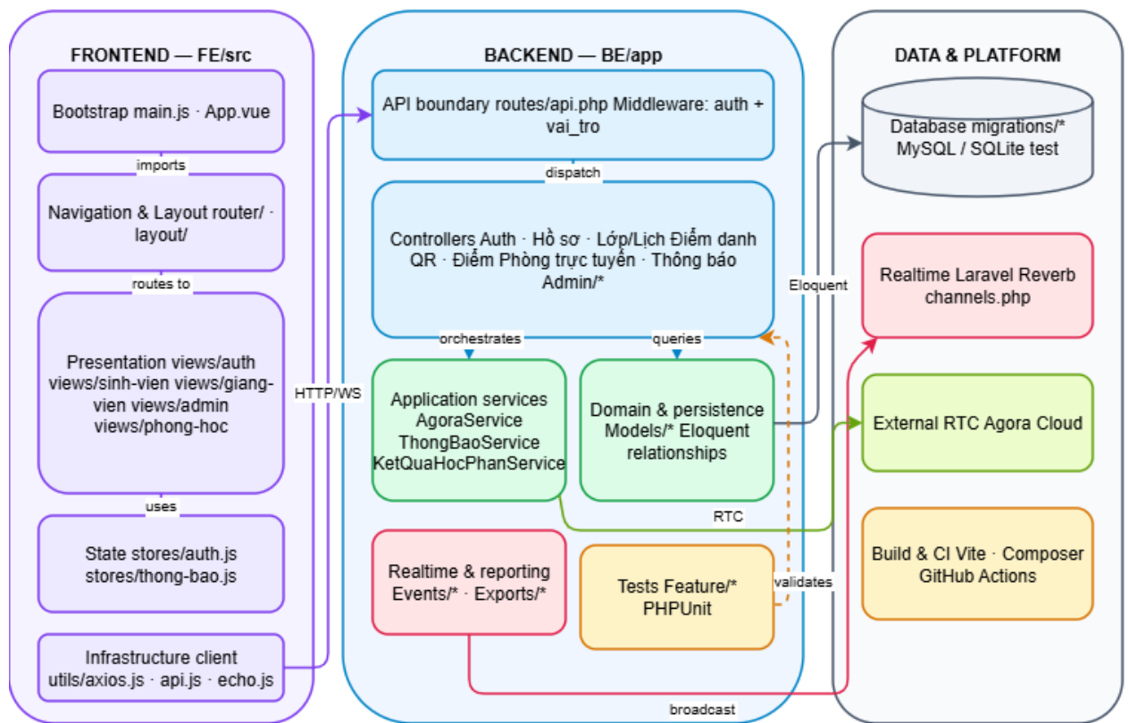
Hình 3: Module view
