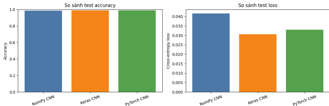
Hình 8: Biểu đồ đối chiếu Test Accuracy và Test Loss trên 10,000 ảnh kiểm thử MNIST
