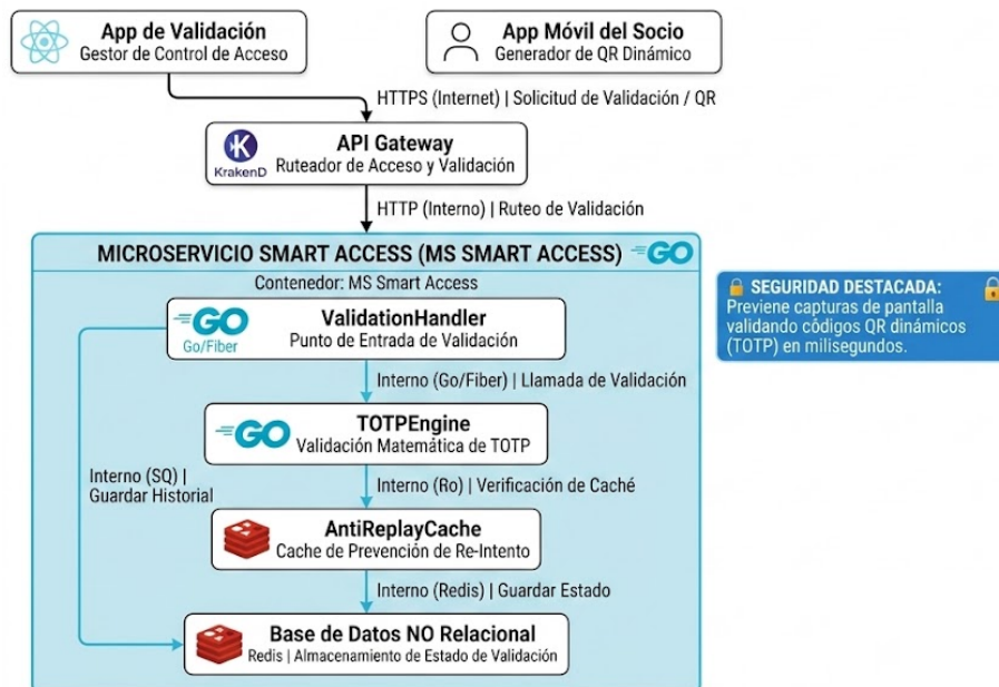
Figura 6: Diagrama C4 nivel 3: Componentes (Microservicio de Acceso Inteligente). Lógica interna de validación matemática y fuera de línea (offline) mediante contraseñas de un solo uso basadas en el tiempo (TOTP) para el control de acceso en estadios.
