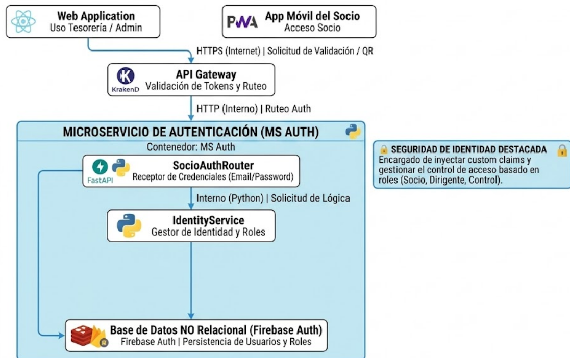
Figura 7: Diagrama C4 nivel 3: Componentes (Microservicio de autenticación). Sistema centralizado para el manejo de identidades, validación de credenciales y generación de vales web JSON (Tokens JWT).
