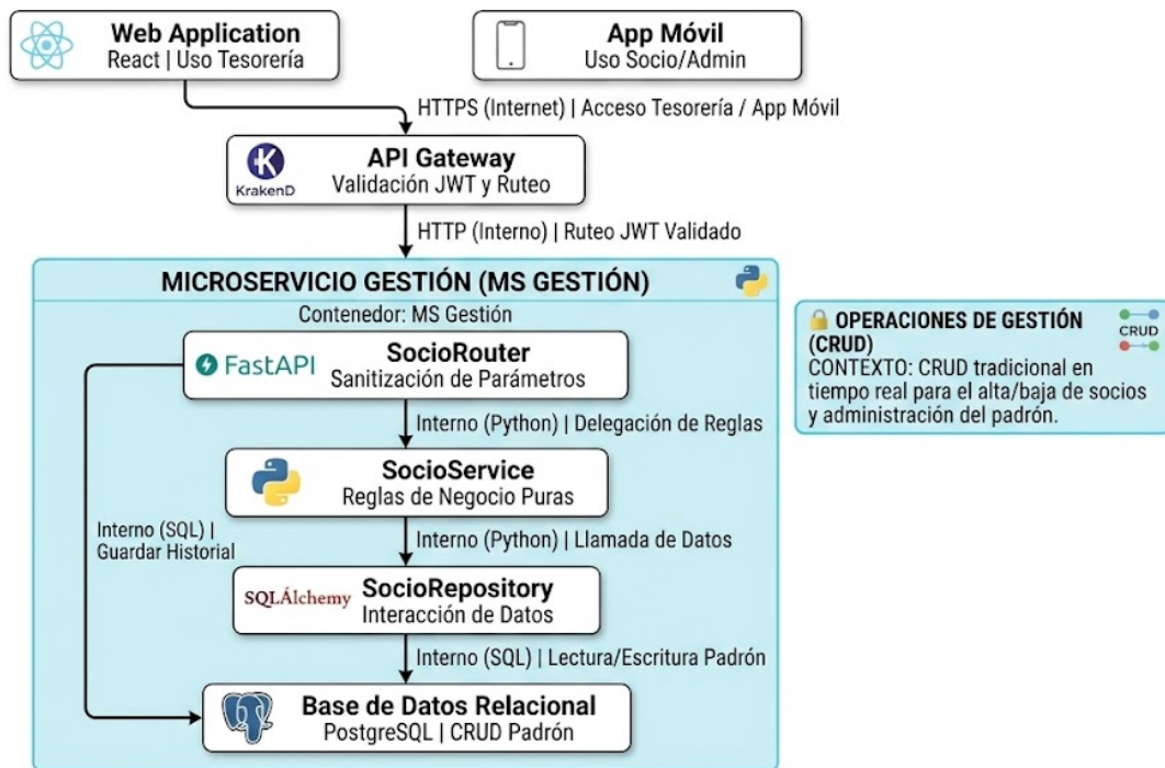
Figura 3: Diagrama C4 nivel 3: Componentes (Microservicio de gestión societaria). Detalle del microservicio principal encargado de la creación, lectura, actualización y borrado (CRUD) de usuarios, perfiles y reglas de negocio del padrón societario.
