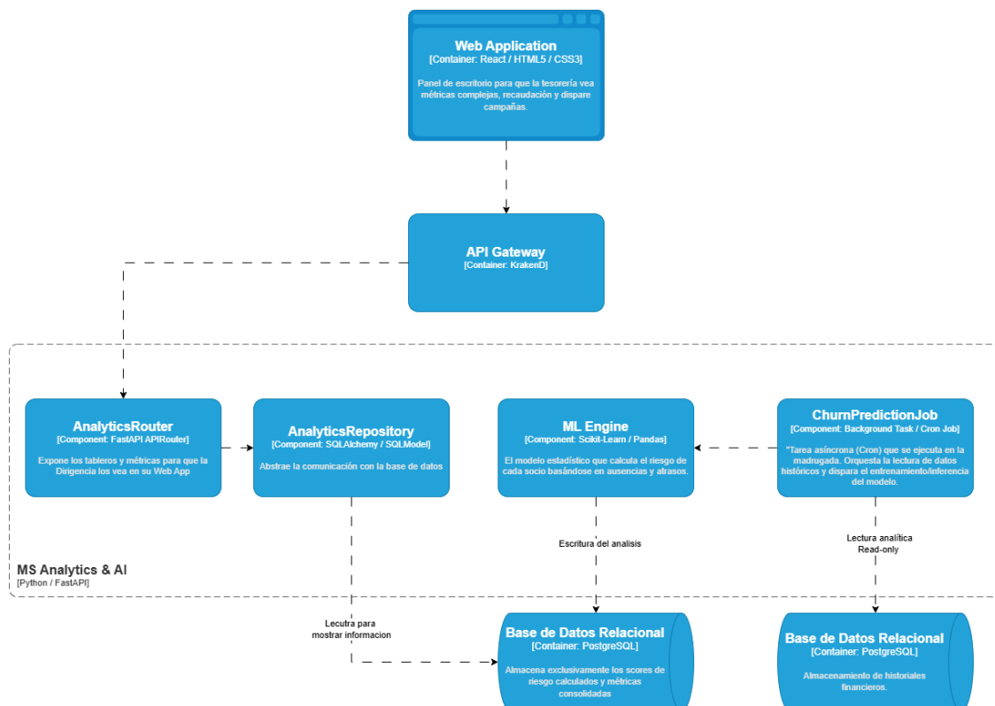
Figura 8: Diagrama C4 nivel 3: Componentes (Microservicio de analytics e inteligencia artificial). Orquestación de tareas asíncronas y motor de Machine Learning para la predicción de riesgo de morosidad.
