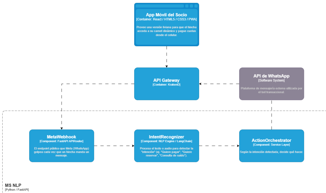
Figura 4: Diagrama C4 nivel 3: Componentes (Microservicio de Procesamiento de Lenguaje Natural [PLN]). Detalle del motor de procesamiento de lenguaje natural integrado vía retrollamada web (Webhook) con la API de WhatsApp para la atención automatizada.
