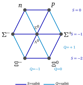
Baryon Okteti — 1961
