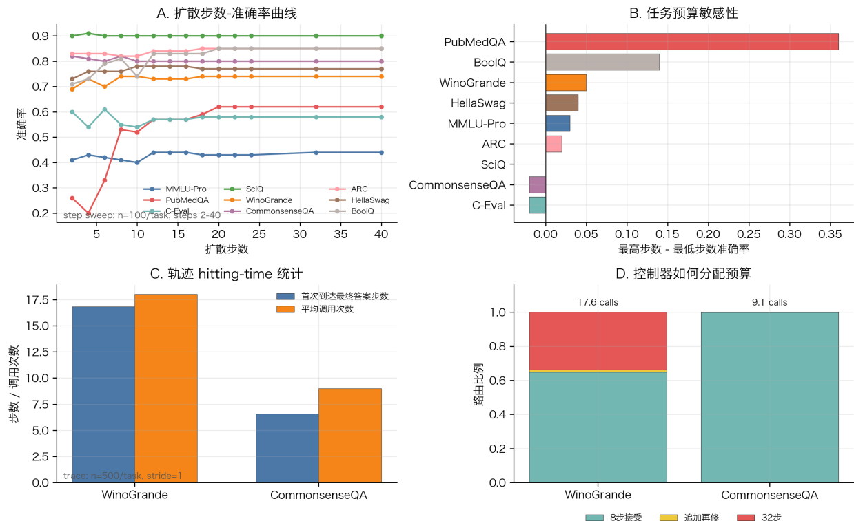
推理侧证据合图：步数曲线、轨迹稳定性与预算路由
