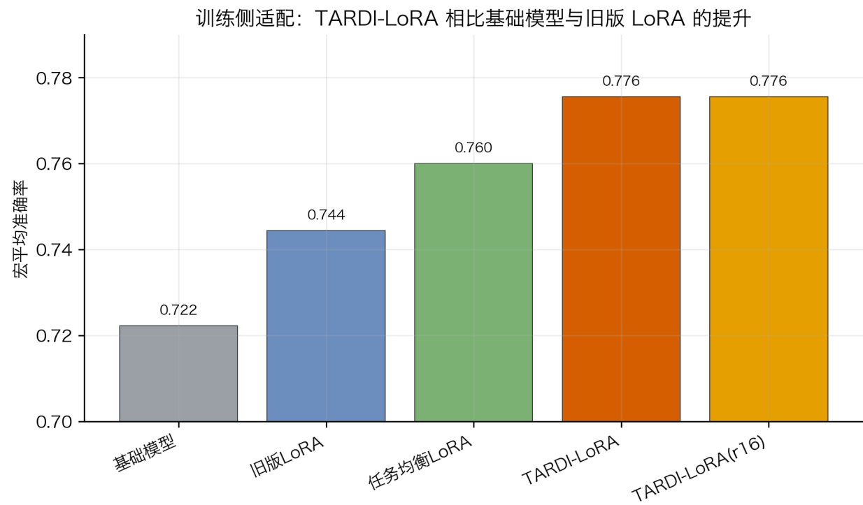
图 1 展示了训练侧主要消融。基础 LLaDA 在 9 个任务上的宏平均准确率为 0.722。旧版 LoRA 达到 0.744。仅做任务均衡后提升到 0.760。加入高噪声终标签去噪后，TARDI-LoRA 达到 0.776，与 r16 配置相同。
