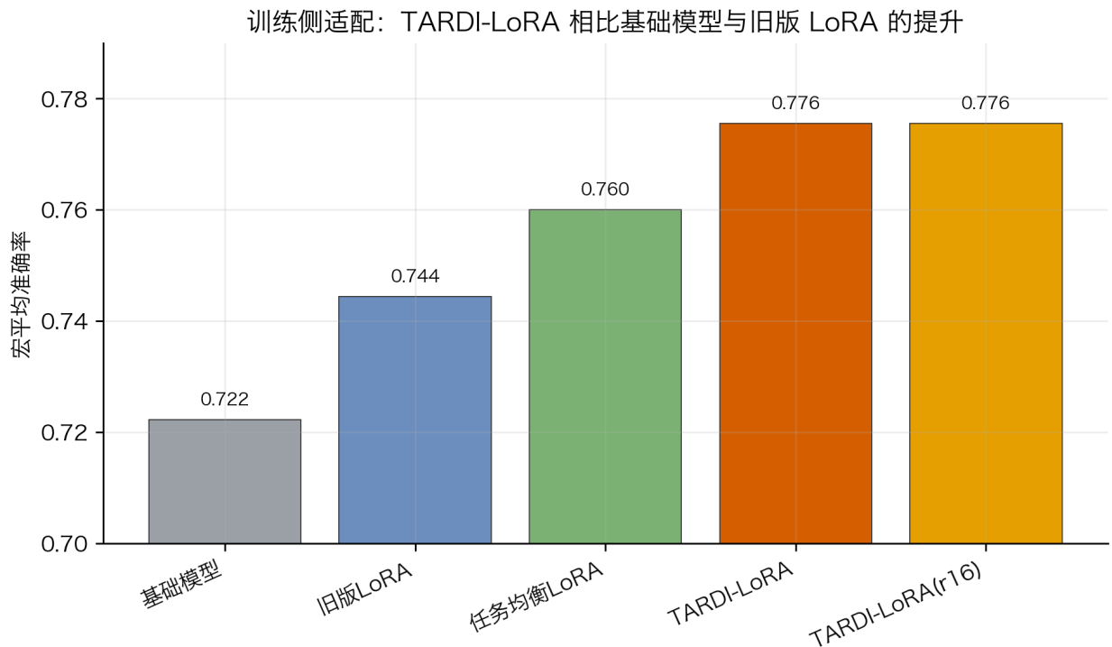
Figure 2: 训练侧 LoRA 主结果
