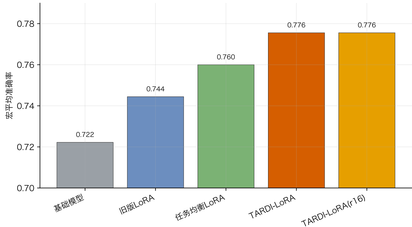
训练侧适配：TARDI-LoRA 相比基础模型与旧版 LoRA 的提升
